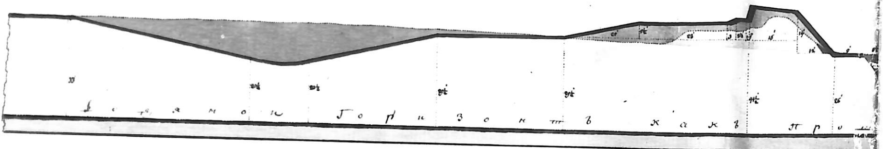
№ 8. Профиль правого зема нарж го полигона курткины.
