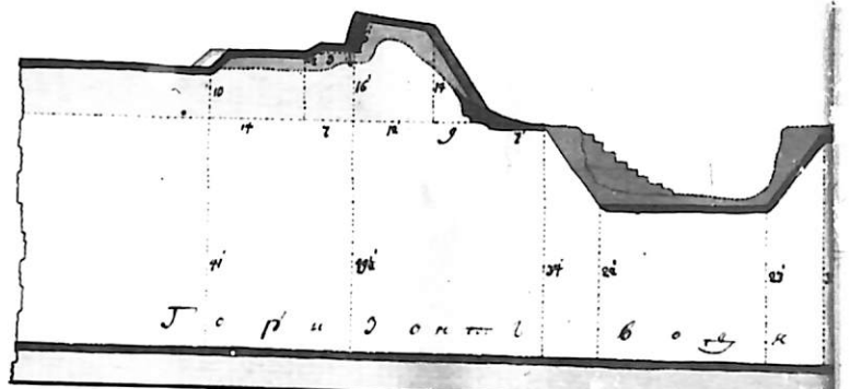
№ 9. Профиль чрез левый фланг 6 го ватикона
